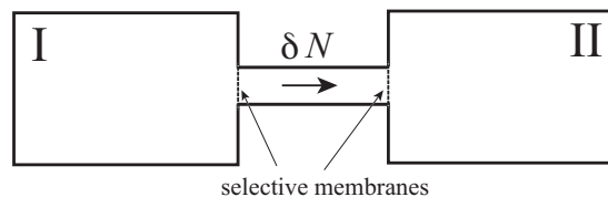
Figure 16.1: 二つの系は，今考えている目的化学物質だけを選択的に透過させる膜を介して接触している．図の真ん中の結合部分には不要であるが，目的化合物だけが交換されていることをはっきりさせるために入れてある（しかし，単離できない化合物はいっぱいあることを忘れるべきでない → 25.6）．
