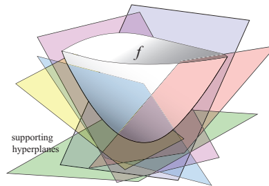
Figure C.1: f の支持超平面の例
