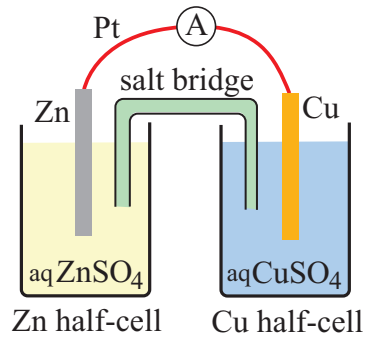
Figure 26.8: Daniell 電池
