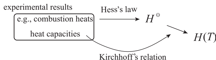
Figure 25.3: どうやって標準エンタルピーを測定できる量から決めるか; まとめ
