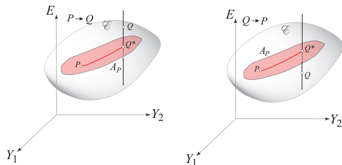
Figure B.1: 左: P から Q^* には断熱的に行ける。もしも Q^* が Q より小さな内部エネルギーを持っているならば Q^* から Q に垂直に (断熱不可逆的に) 行くことができる。右: もしも Q が Q^* より下にあると、断熱的に Q^* から Q に行くことはできない。しかし、断熱的に Q から Q^* にはいける。 P - Q^* は可逆なので Q から P へ断熱的に行ける。
